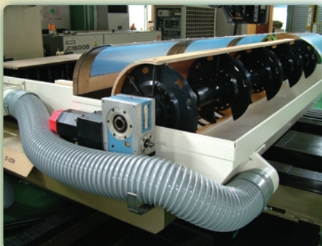
ロータリー兼用型レーザー加工機
